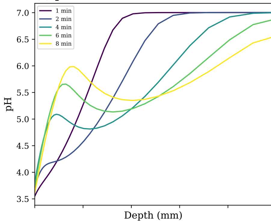
(d) \text{H}_2\text{O}_2
