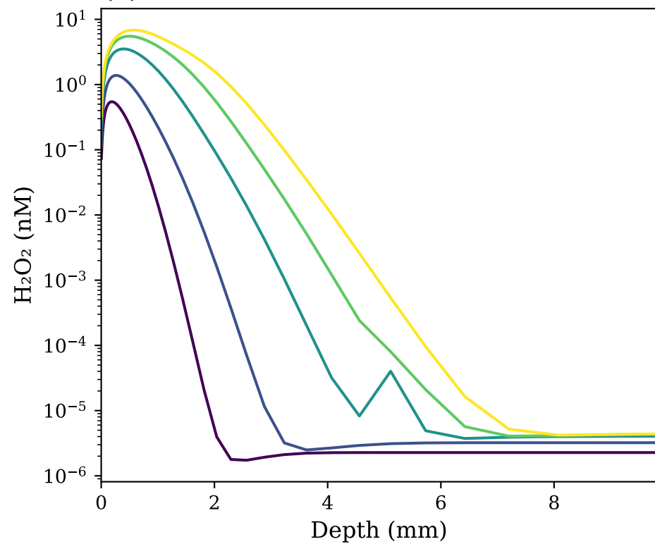
(d) \text{H}_2\text{O}_2
